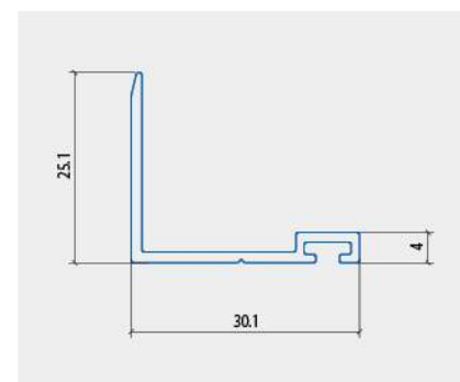
ỐP ĐỨNG CÁNH LÙA 1 RAY
