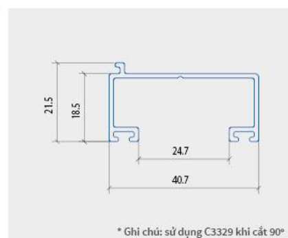
ỐP CHÂN CỬA ĐI
