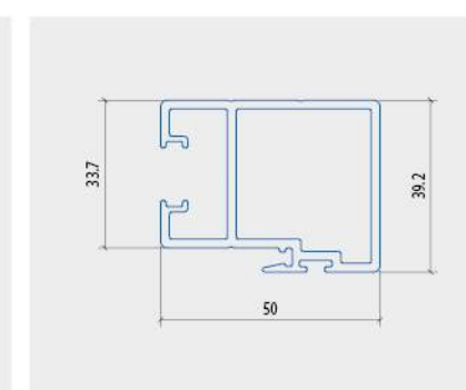
THANH ĐỨNG CẢNH MÓC
