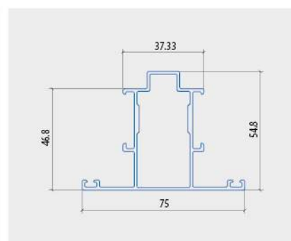
ĐỖ CHỮ T CHO KHUNG BAO
