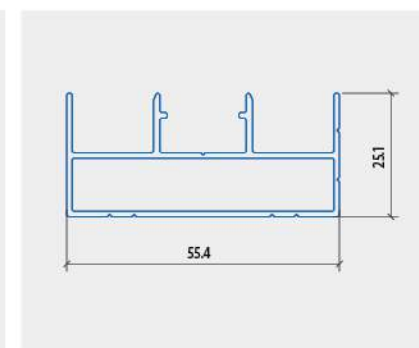
ĐỨNG KB LÙA 1 RAY
