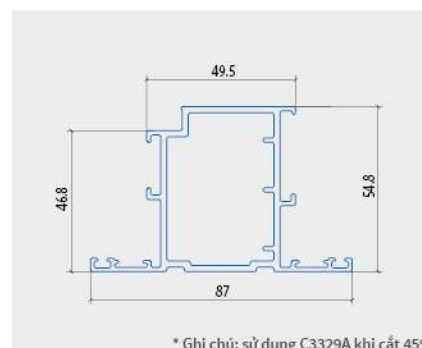
CÁNH CỬA ĐI MỞ NGOÀI
