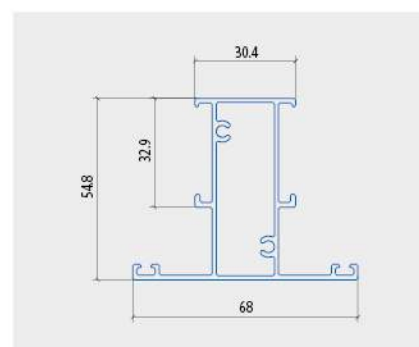
ĐỖ CHỮ T CHO CÁNH
