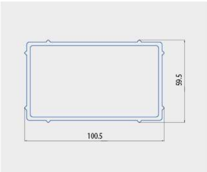
NÒNG NỐI MD651
