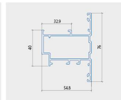
CÁNH CỬA SỔ
