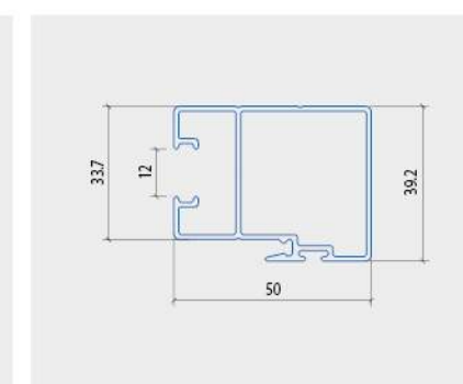
THANH ĐỨNG CẢNH MÓC
