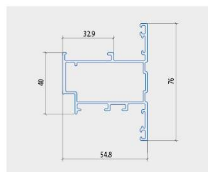
CÁNH CỬA SỔ (Mã dùng riêng)
