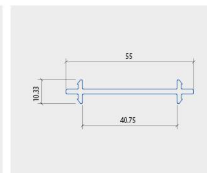
NỆP NỔI KHUNG
