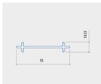
NẠP NỐI KHUNG
