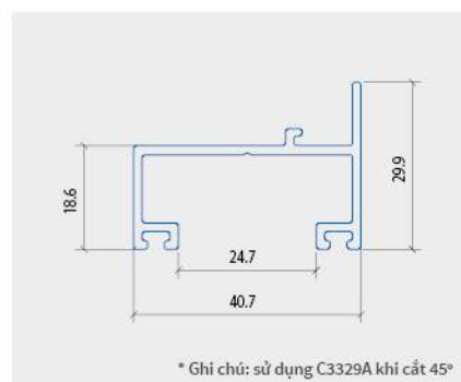
ỐP CHÂN CỬA ĐI
