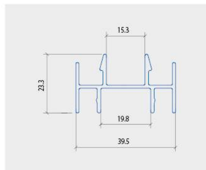
THANH ỐP ĐỐI ĐẦU 4 CẢNH
