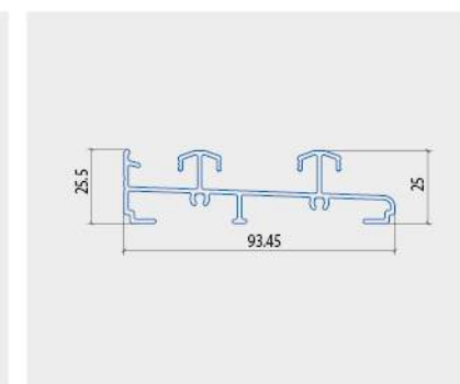
RAY TRÊN DƯỚI
