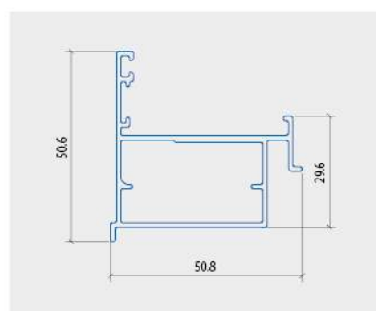
NẠP CHUYỂN HƯỚNG CHIẾU MỜ
