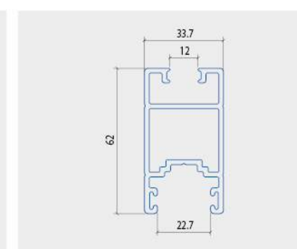
THANH ĐỨNG CẢNH
