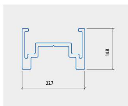
NẾP CHO KÍNH HỘP CỬA TRƯỢT
