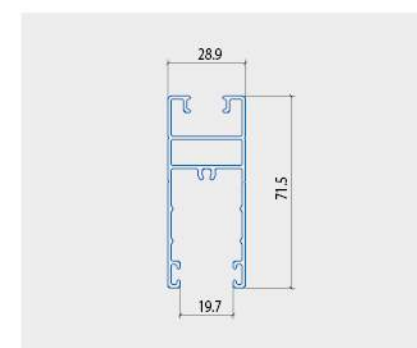
THANH NGANG CẢNH DƯỚI
