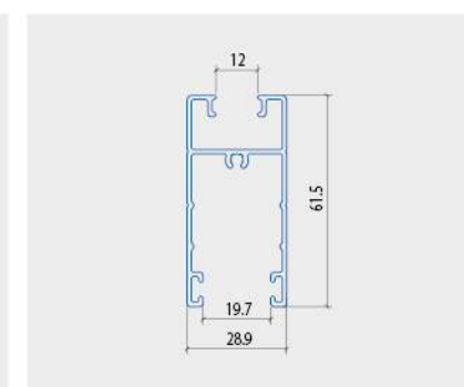
THANH NGANG CẢNH DƯỚI
