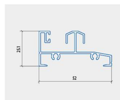
NGANG RAY DƯỚI LÙA 1 RAY
