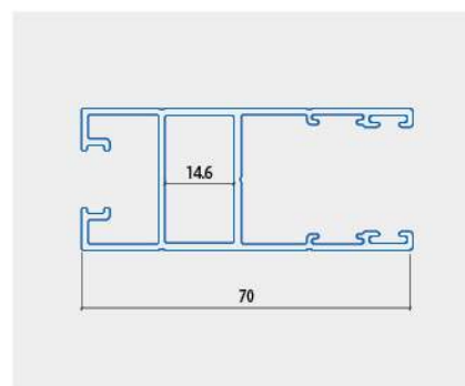
KHUNG CÁNH CỬA TRƯỢT 55
