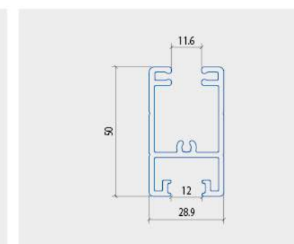
NGANG CẢNH TRÊN
