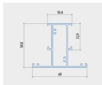
ĐỖ CHỮ T CHO CÁNH
